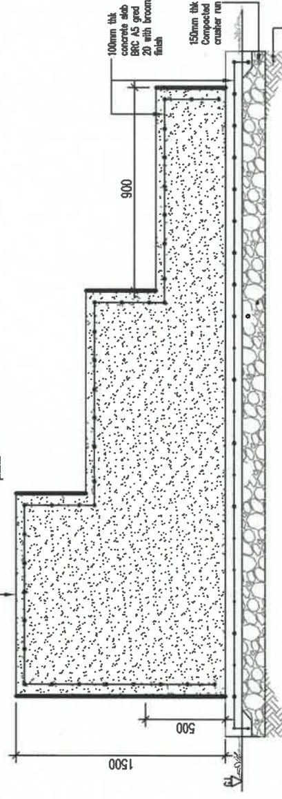
KERATAN A-A
