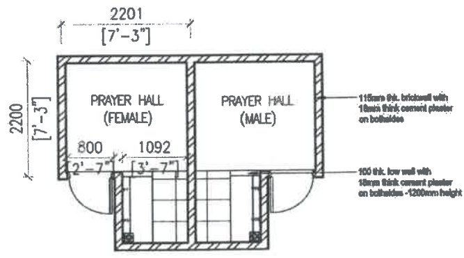
Rajah 5.3 : Pelan Lantai Ruang Solat Bagi 14'x 7'
