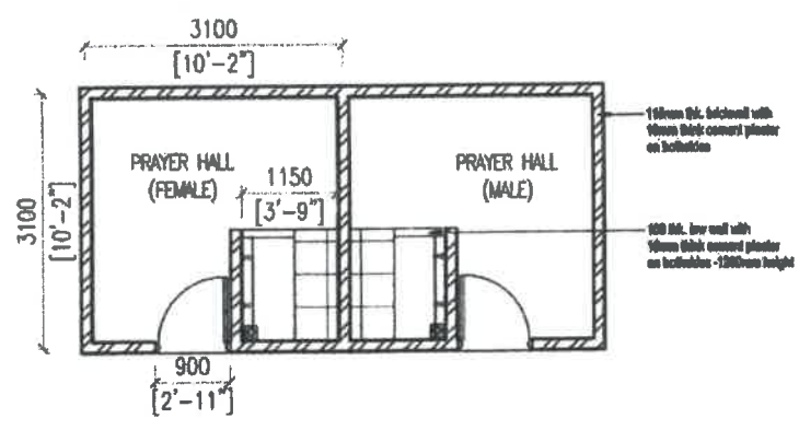
Rajah 5.2 : Pelan Lantai Ruang Solat Bagi 20'x 10'
